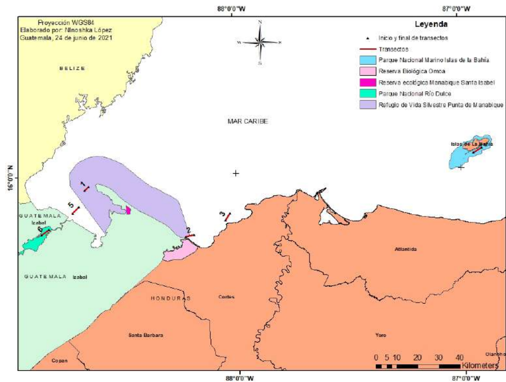
Figura 1. Transectos de arrastre para colecta de muestras de microplásticos durante expedición Plasticósfera. Los números de transectos corresponden a la siguiente manera: (1) Refugio de Vida Silvestre (RVS) Punta de Manabique, (2) Desembocadura de Motagua, (3) Omoa, (4) Parque Nacional (PN) Utila, (5) Bahía de Amatique y (6) PN Río Dulce.
